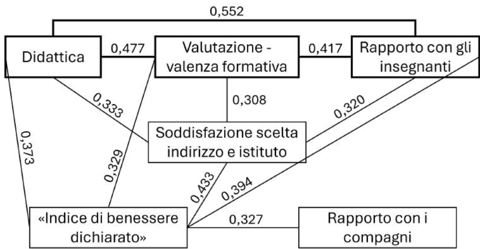
Fig. 3: Correlazioni salienti tra diverse dimensioni del benessere a scuola (coefficiente di Tau b di Kendall, p < 0,001 )
