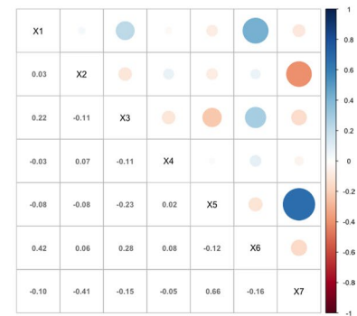
(d) Cluster 4
