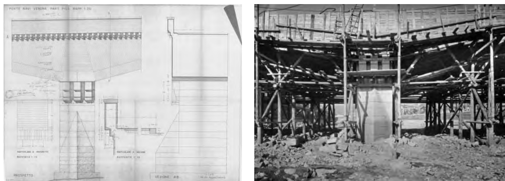
Fig. 5 – Ricostruzione di ponte delle Navi, 1947-49: dettaglio architettonico della pila (BCVr) e vista del cantiere durante i lavori (ASVr).
