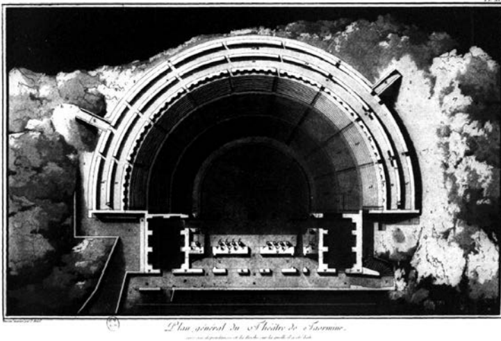
Fig. 3 ~ Jean-Pierre Houel, Pianta del teatro di Taormina (HOUEL 1782-87, tav. 94).
