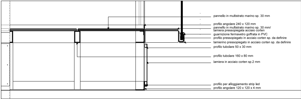
IL PRESEPE FAVOLOSO | TECA | Disegni Esecutivi | Sezione B-B' | scala 1:10
